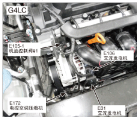
18. 发动机左侧
