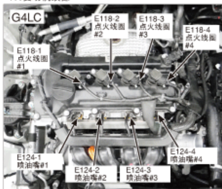
17. 发动机顶部
